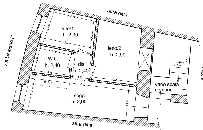
Piano Primo 1:100 porzione 2/2
