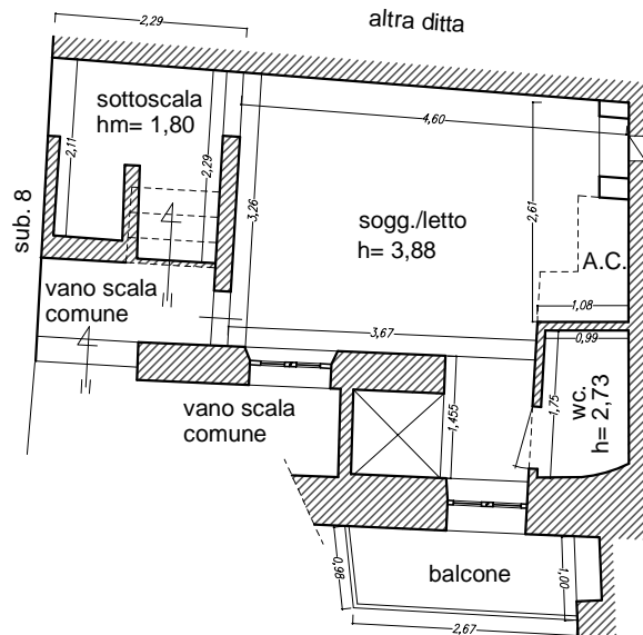
Piano Primo 1:100 porzione 1/2
