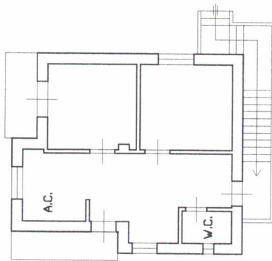
Planta Piano Primo Abitazione int.2 H= 2,80m
