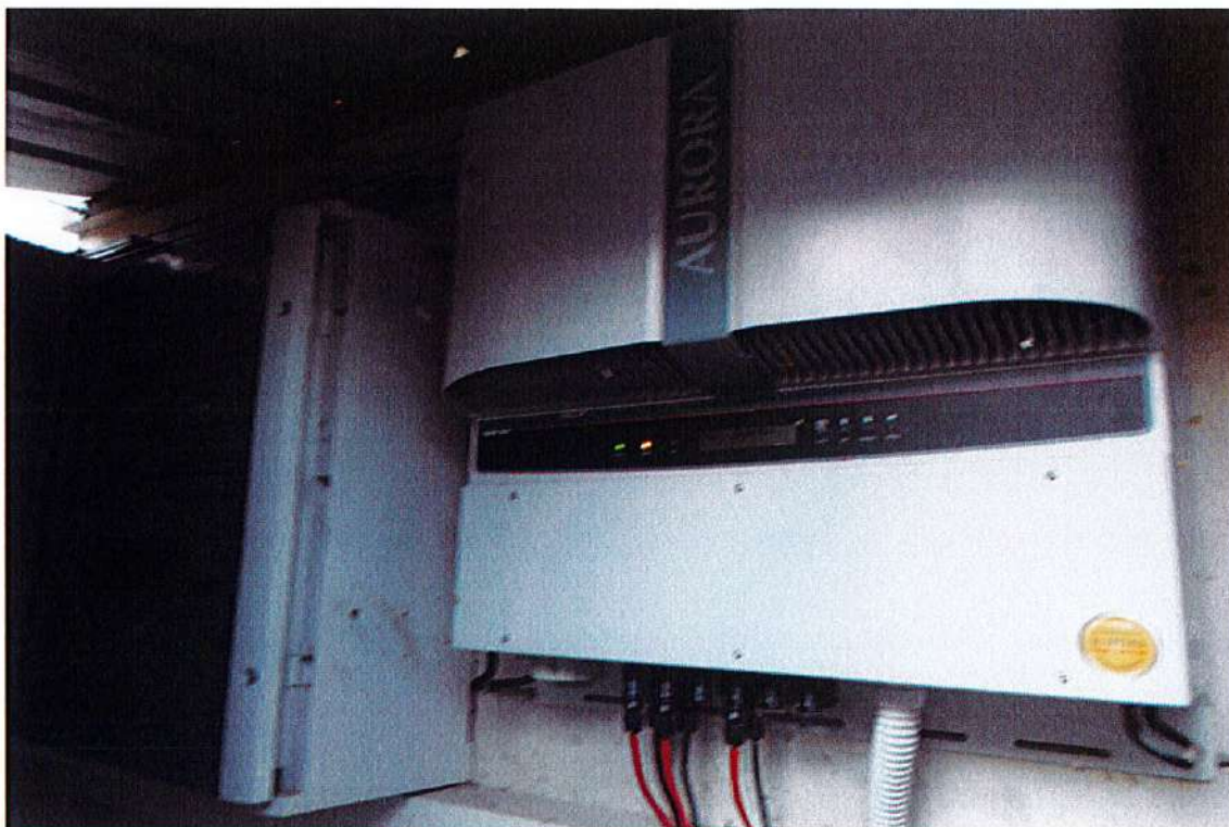
Particolare inverte e quadro elettrico
