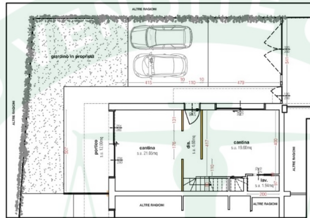
LEGENDA DIVISORI MANCANTI PLANIMETRIA PIANO SEMINTERRATO H=2,60m
