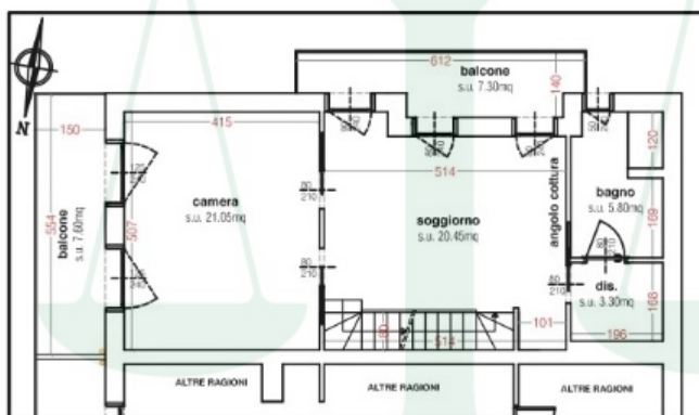
PLANIMETRIA PIANO RIALZATO (da licenza edilizia SCIA n. 2166/2013) H=2,70m
