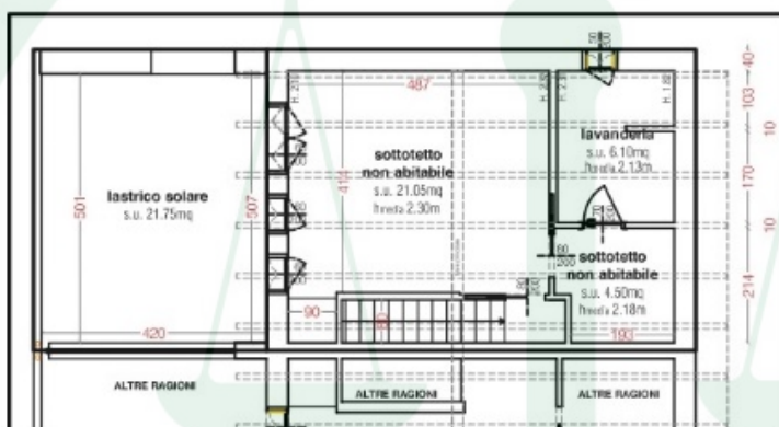
PLANIMETRIA PIANO PRIMO SOTTOTETTO (da licenza edilizia SCIA n. 2166/2013)
