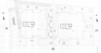
Pianta copertura - scala 1:100
