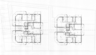
Pianta piano secondo - scala 1:100
