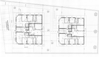
Pianta piano rialzato - scala 1:100
