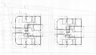
Pianta piano primo - scala 1:100
