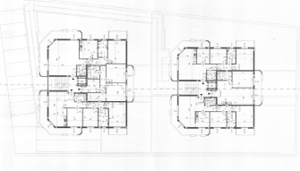
Pianta piano terzo - scala 1:100
