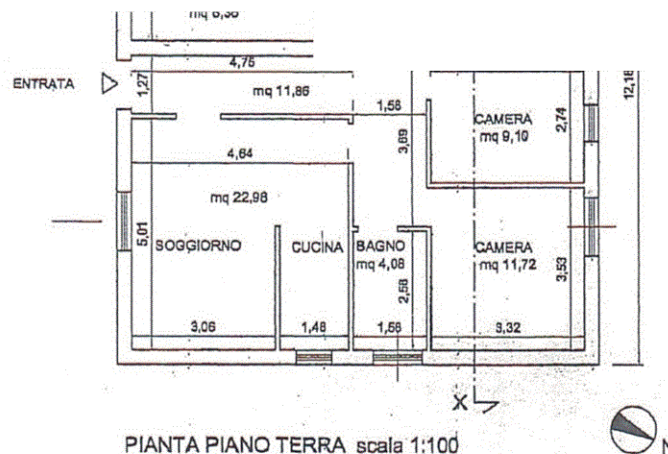
Planimetria di progetto in sanatoria
