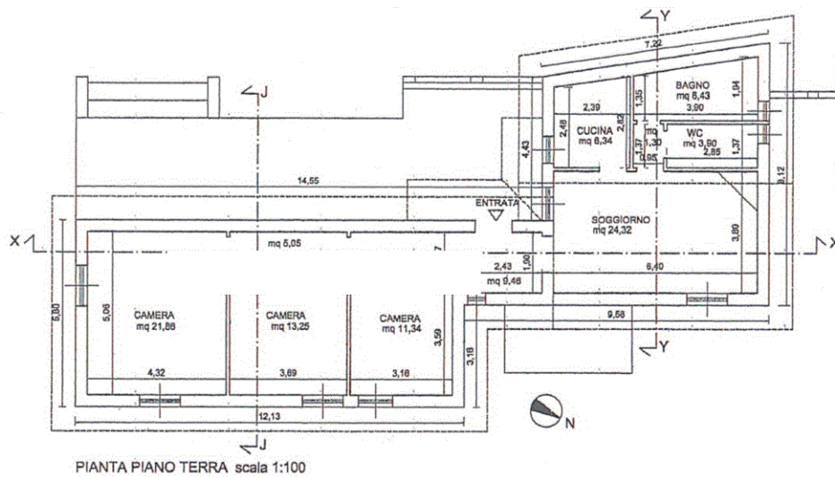
Planimetria di progetto in sanatoria
