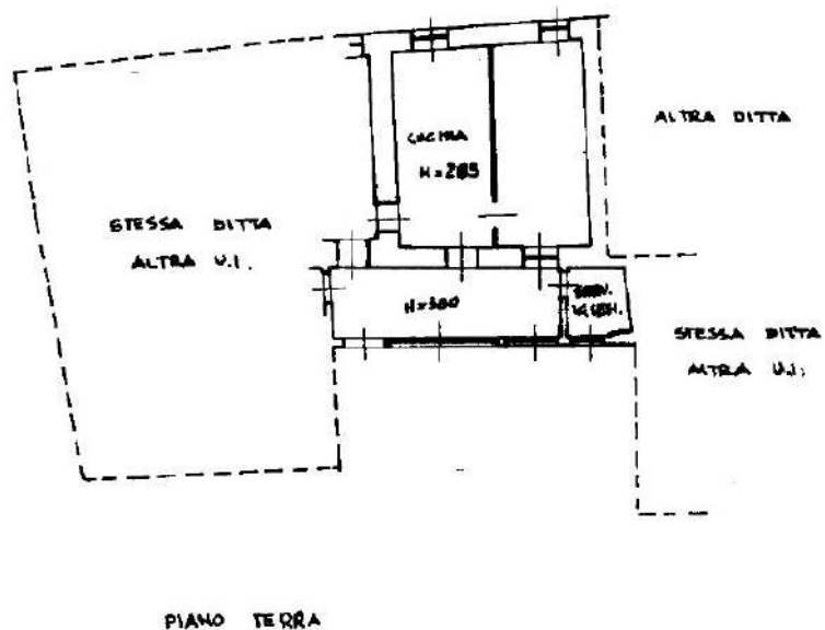
Planimetrie piano terra e primo
