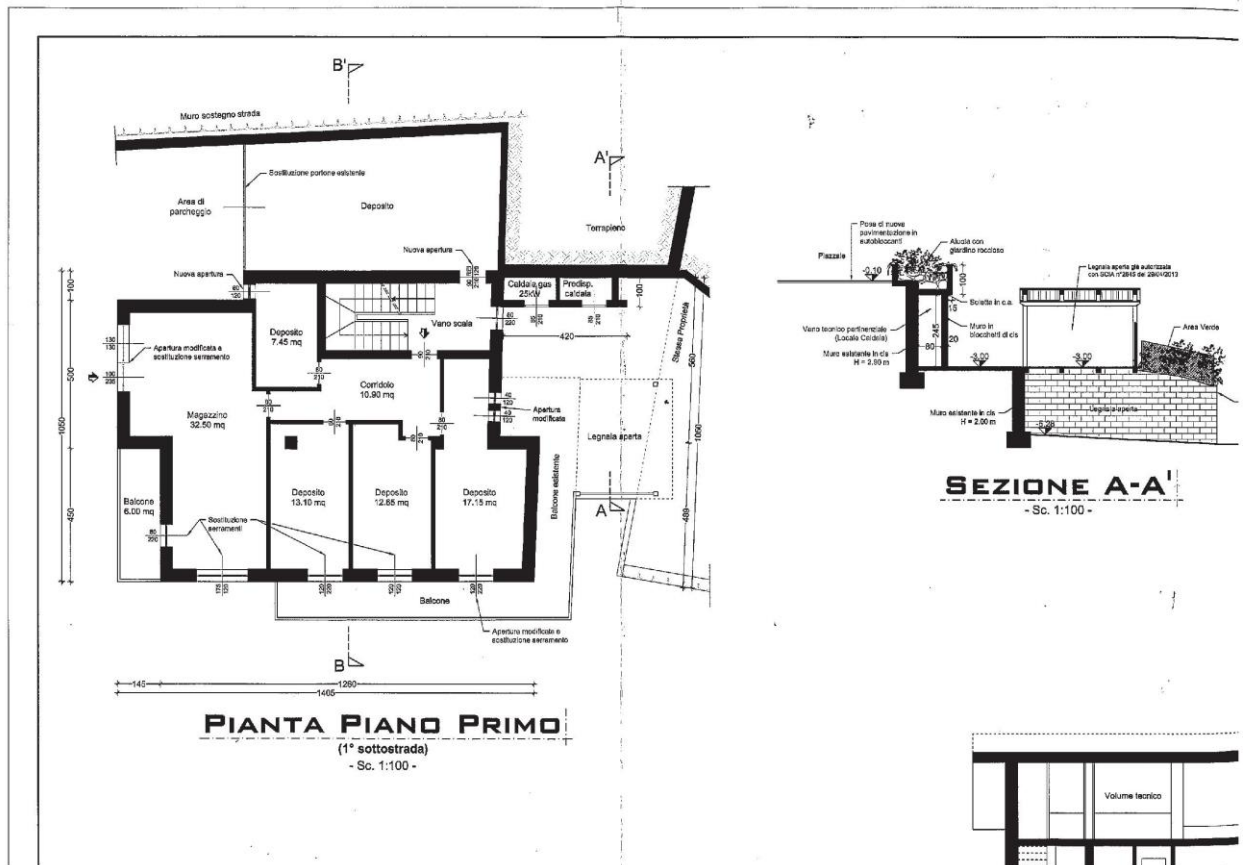
PLANIMETRIA MAGAZZINO-ALLOGGIO IN CORSO DI COSTRUZIONE AL PIANO 1° SEMINTERRATO
