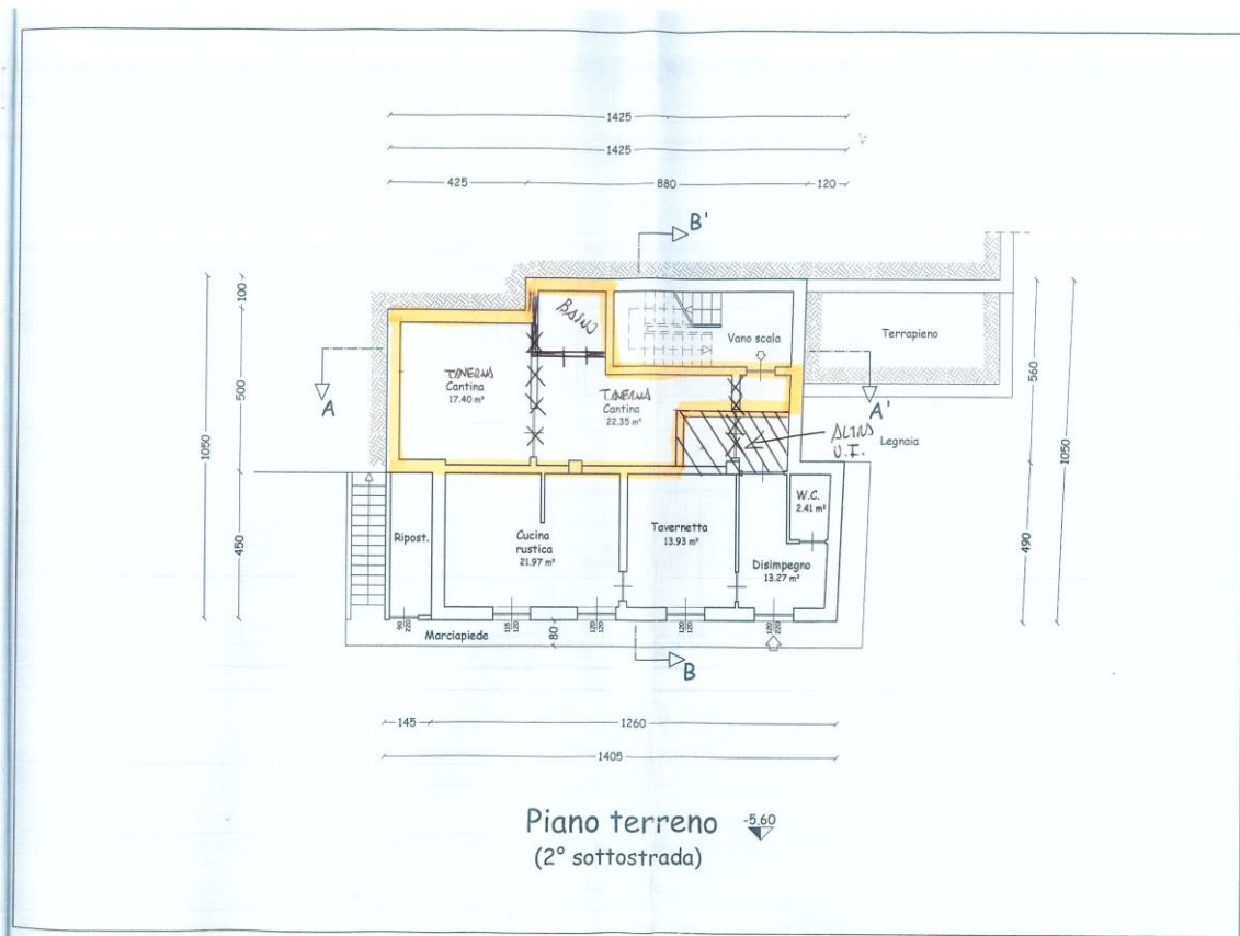
CANTINA-TAVERNA AL PIANO 2° SEMINTERRATO CON ALCUNI PARTICOLARI AGGIUNTI INDICATIVI DELLO STATO DI FATTO.
