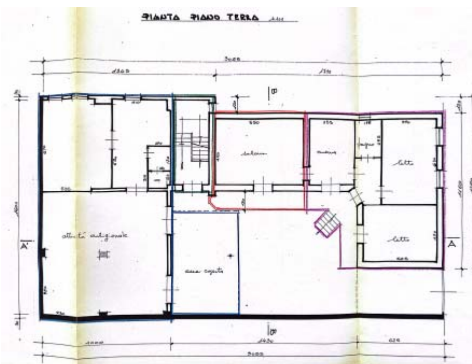
Stralcio relativo al piano terra, tratto dai grafici a corredo della pratica di condono prot. 10360/86 (sulla sinistra, bordato in blu, il locale per attività artigianale)
