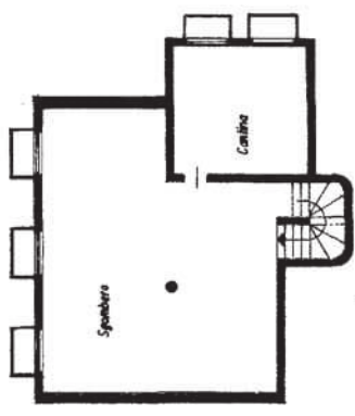
Piano Primo Sottosopra h=2,40
