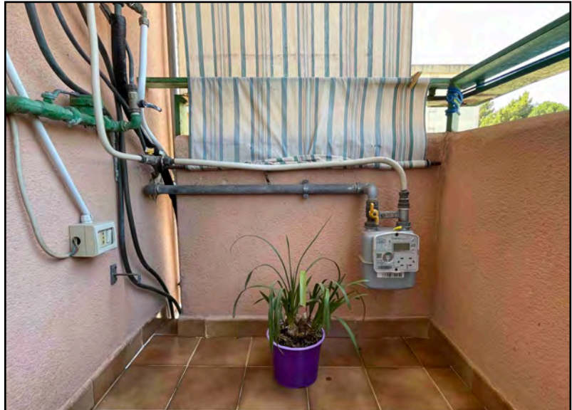
Impianto del gas
