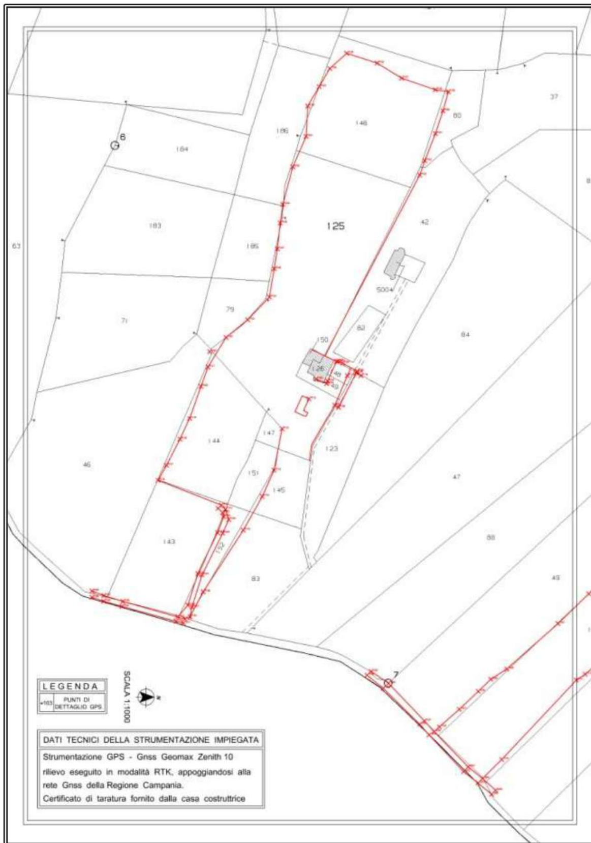
Figura 18 rilievo topografico
