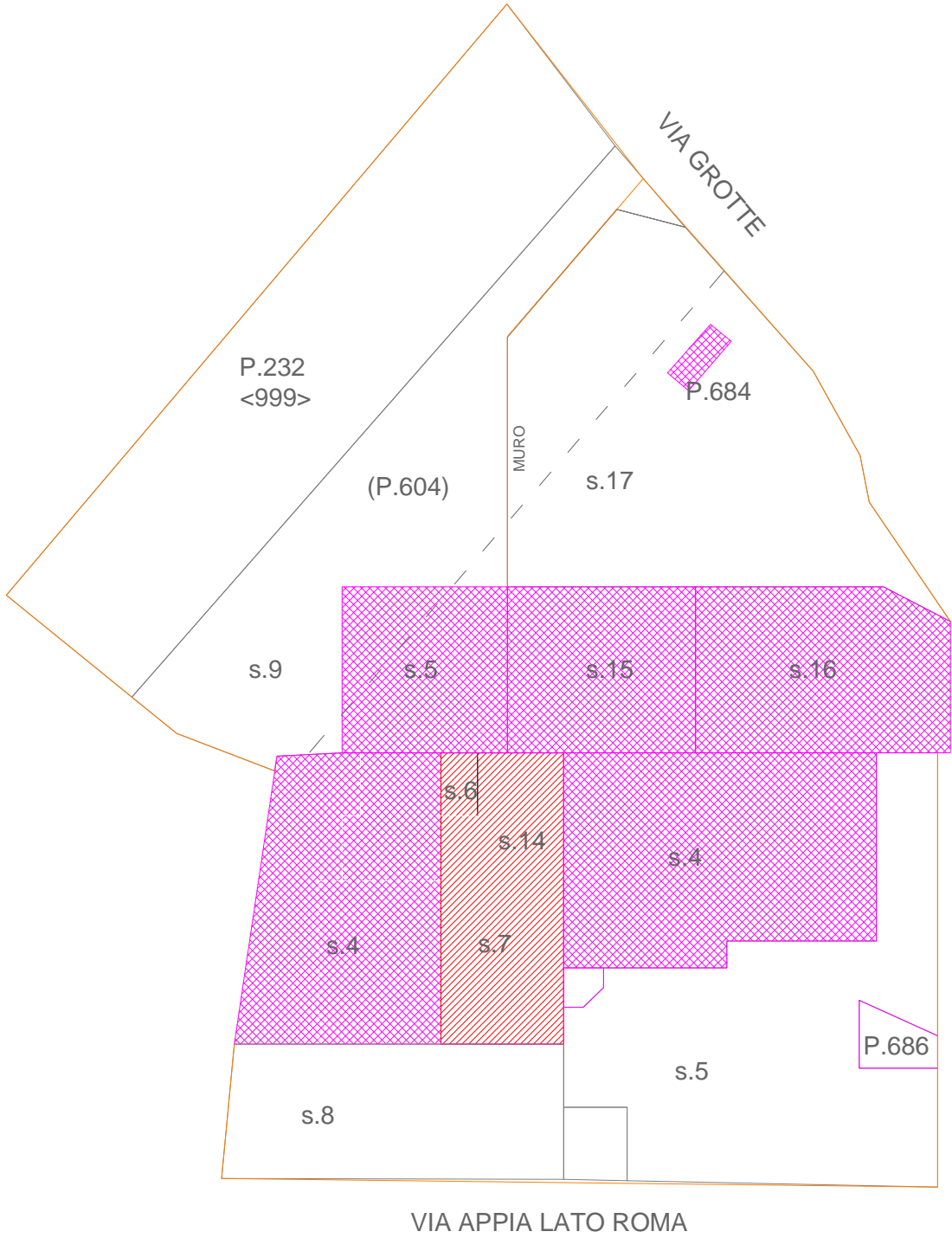
Planimetria dei diversi sub contenuti nel complesso industriale
