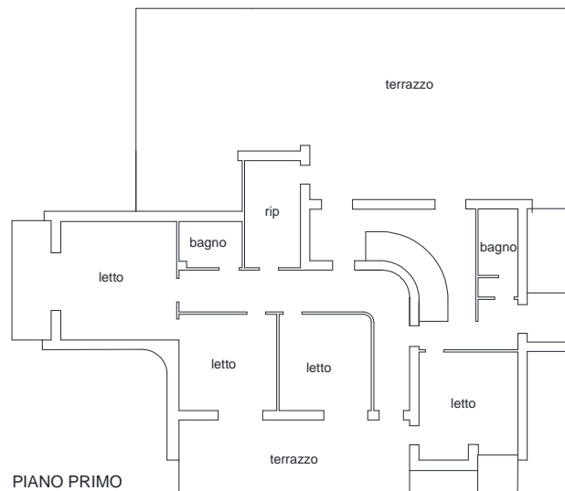
Villino. Pianta piano primo
