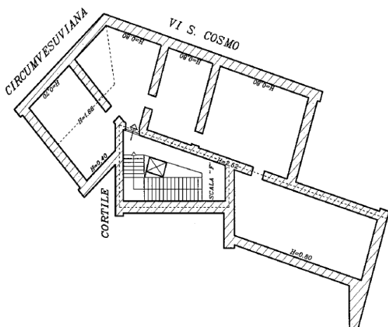
Grafico n. 3 - Planimetria del sottotetto sub. 221
