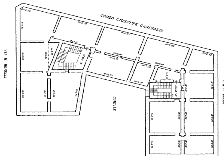
Grafico n. 11 - Planimetria del sottotetto al fg. 10, p.lla 237, sub 48
