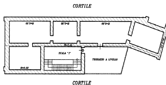
Grafico n. 5 - Planimetria del sottotetto al sub. 224
