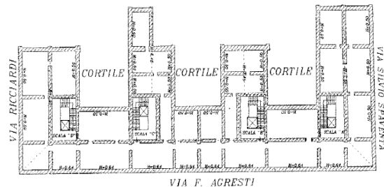
Grafico n. 1 - Planimetria del sottotetto sub. 219
