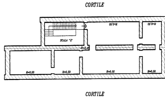
Grafico n. 6 - Planimetria del sottotetto al sub. 225
