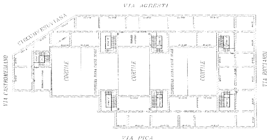
Grafico n. 10 - Planimetria sottotetto al fg. 3, p.la 103, sub. 164
