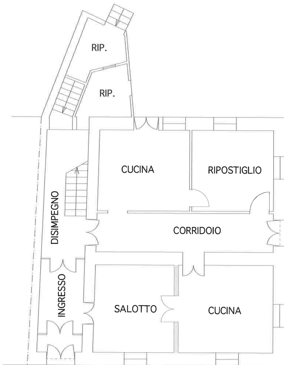
PIANO TERRA Difformità
