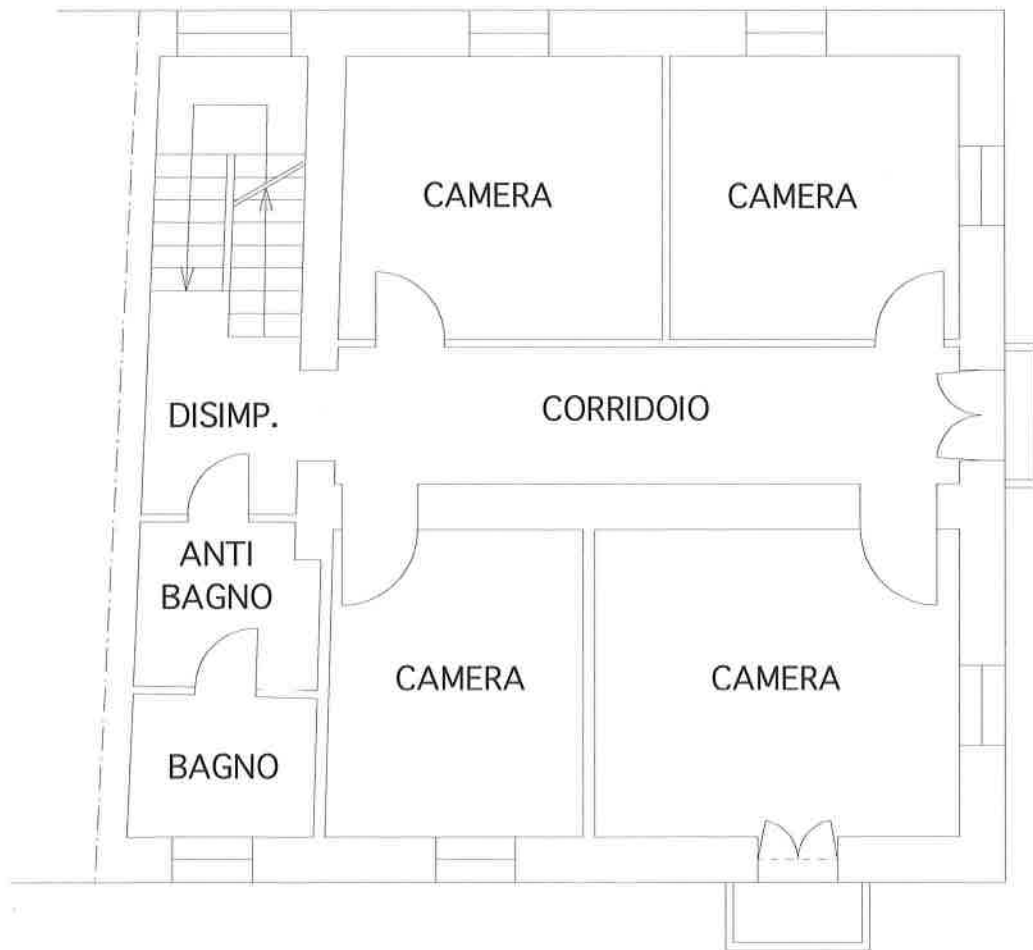
PIANO PRIMO H 275
