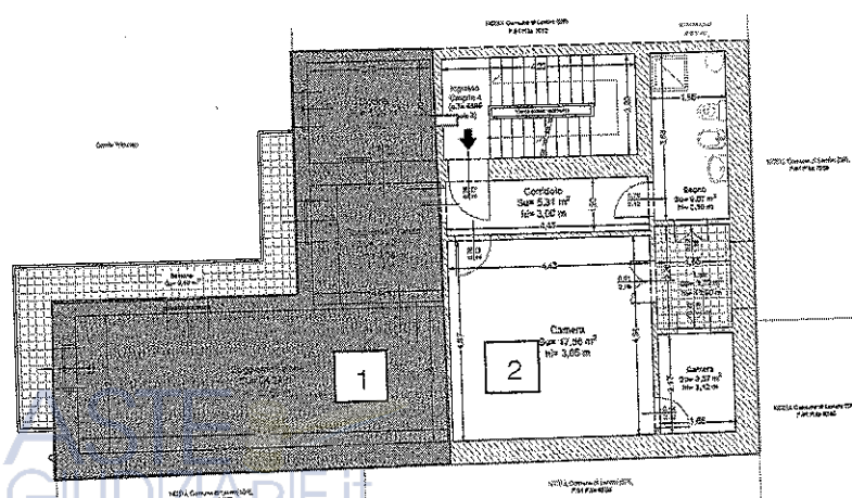
Cespite 4 Appartamento (sub 3) Pianta piano primo - scala 1:100
