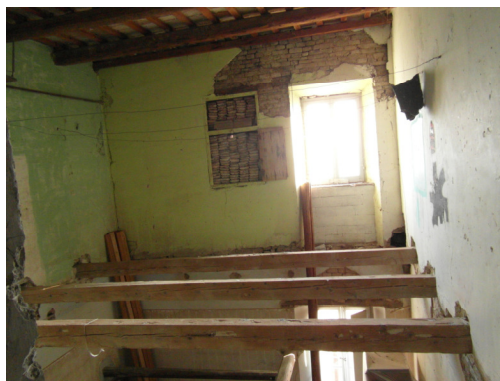
FOTO N. 19 solaio demolito
