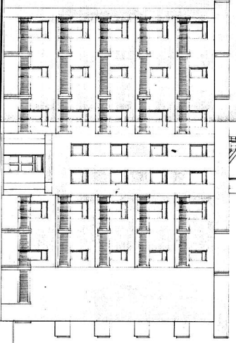
PROSPETTO OVEST
