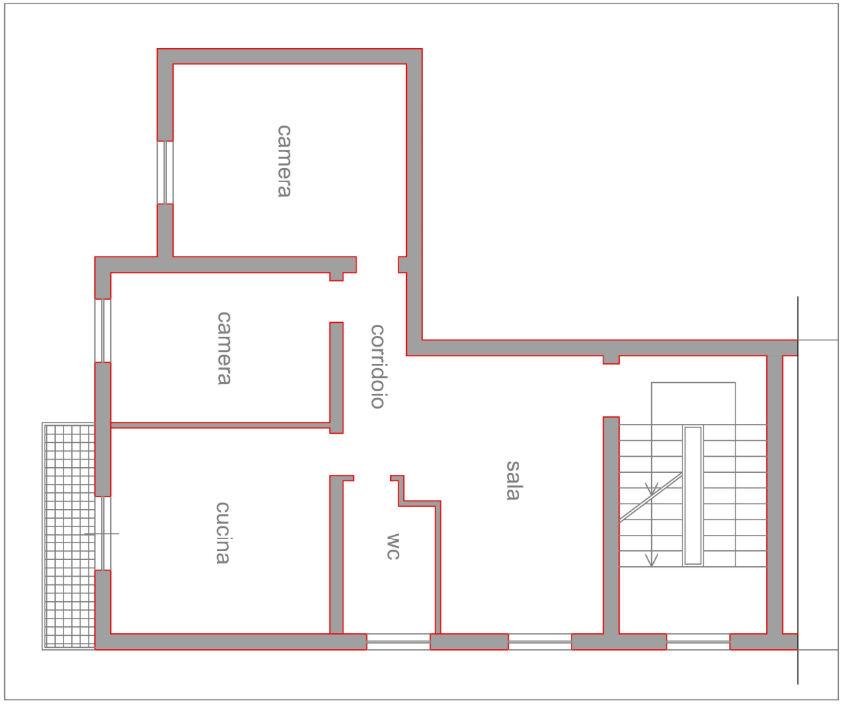
PLANIMETRIA STATO RILEVATO APPARTAMENTO V Sassari n. 135/c P. 3° NCEU Fig. 8 Part. 4345 Sub 7
