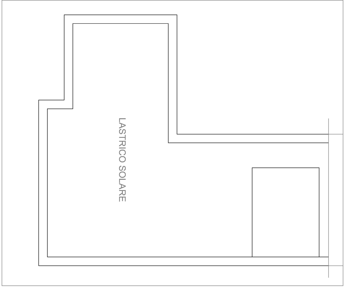
PLANIMETRIA STATO RILEVATO LASTRICO SOLARE V. Sassari n. 135/c P. 4° NCEU Fig. 8 Part. 4345 Sub 1
