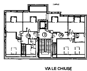
PIANTA PIANO QUARTO (5° F.T.) SOTTOTETTO
