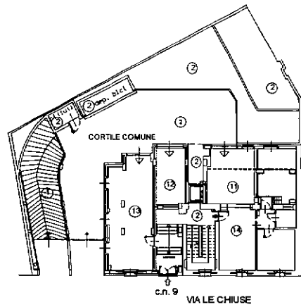
PIANTA PIANO TERRENO (1° F.T.)
